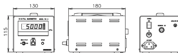
感度切替差圧計 PS-11
