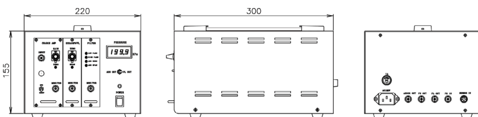
高温用排気圧力計 GCM
